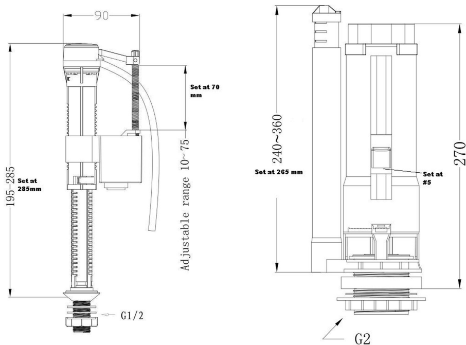
Befolyó szelep
